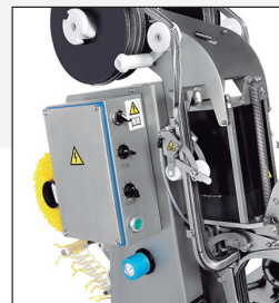
Configuración mediante selectores. Accesorio de clip carrete. Accesorio dispensador de lazos automático.
