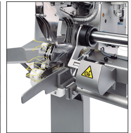
Schwenken des Füllrohrs, um die Zentrierung der Klammer mit minimalem Kraftaufwand zu gewährleisten.
