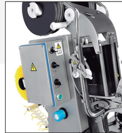
Konfiguration mittels Wahlschalter. Zubehör für Spulenclip. Automatischer Schlaufenspender als Zubehör.
