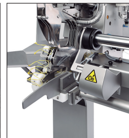
Rotation de tuyau pour centrer le clip avec l'effort minimum / du tube de remplissage afin d'assurer le centrage du clip avec un minimum effort.
