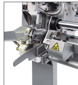
Gir del tub d'embotició per assegurar el centrat del clip amb el mínim esforç.
