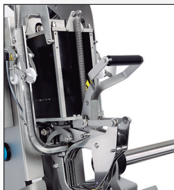
Accionament semi-automàtic de la màquina.
